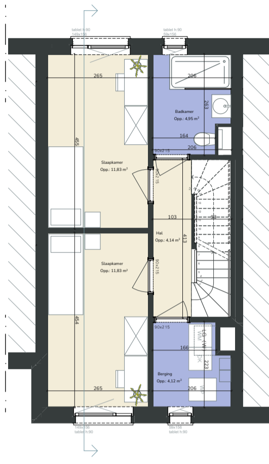
1ste verdieping
