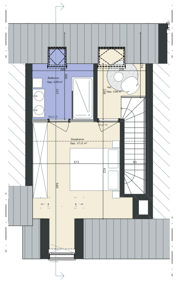
2de verdieping
